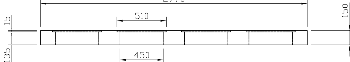
断面図
