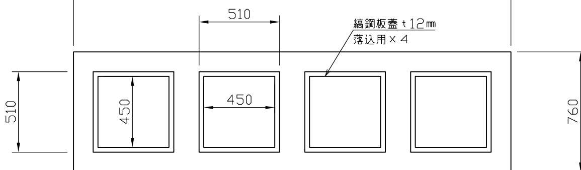
平面図
