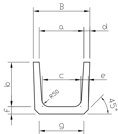
標準断面
