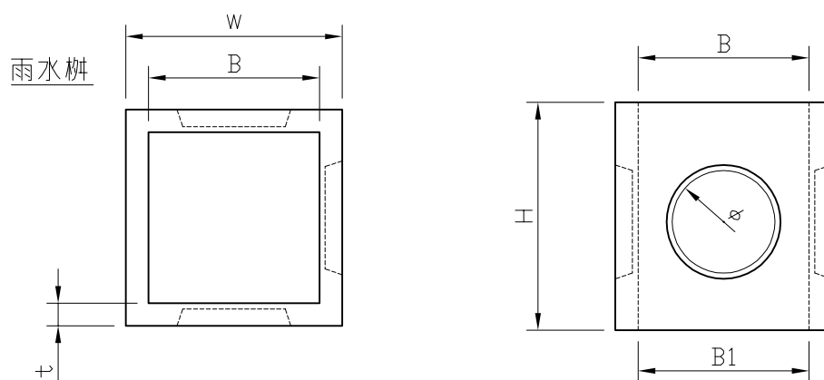
■ マス寸法表
