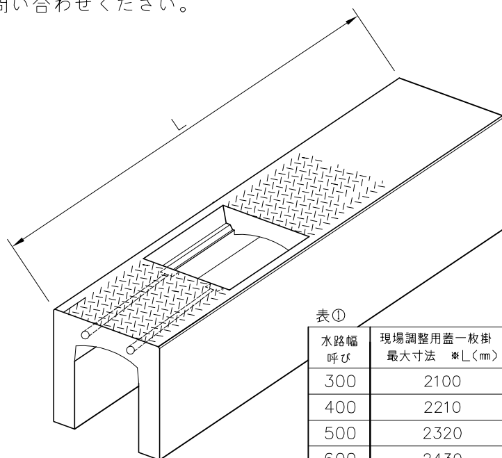
◎現場調整用蓋一枚掛 ご希望の長さにて対応できます。 (L1500~※L)
