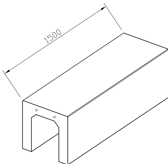
◎暗渠型 ご希望の長さにて対応できます。 (L500~1500)
