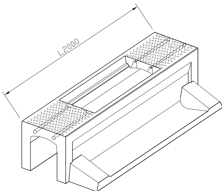
◎土留型 サイズ対応できます。 (水路幅300・400・500・600)
