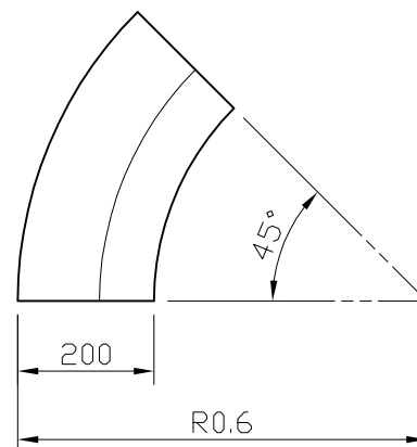
外R0.6 平面図
