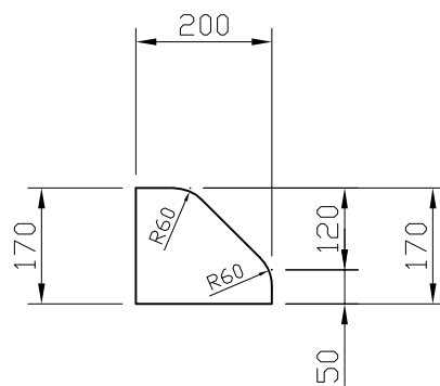
L = 990 正面図
