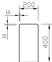
断面図
