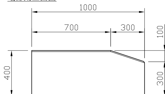
端部用正面図
