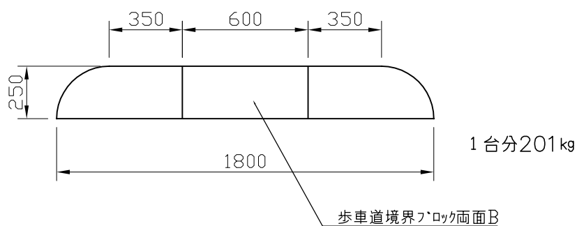
大型車用 正面図
