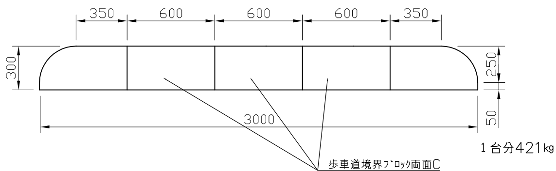
大型車用 正面図
