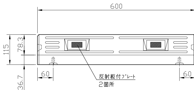
正面図
