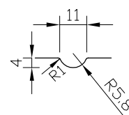
凸模様部詳細図
