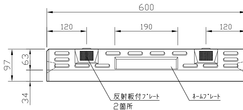
正面図
