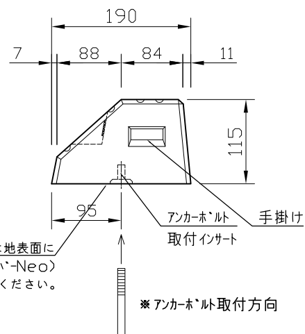
側面図
