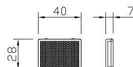
反射板詳細図
