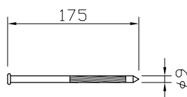
打込アンカーピン詳細図
