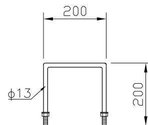
取手金具 溶融亜鉛めっきHDZT 49
