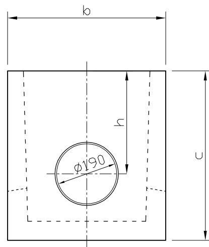
取水方向 断面図
