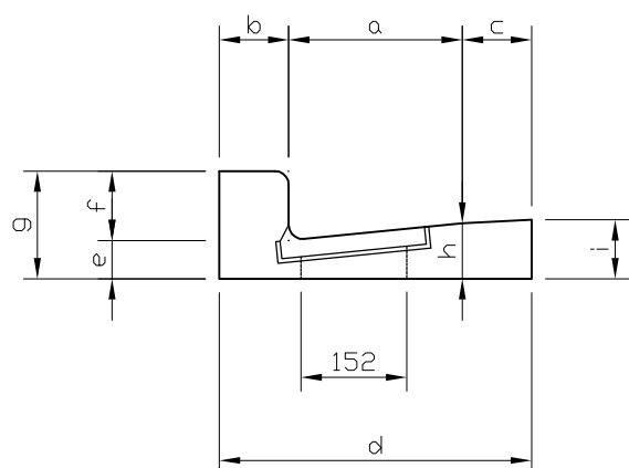
(A-A断面図)
