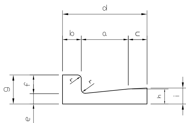
断面図
