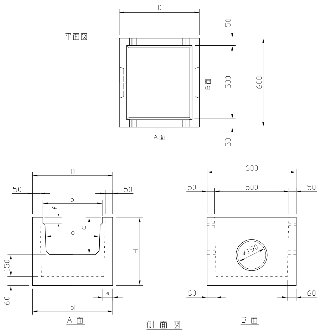
■寸法表
