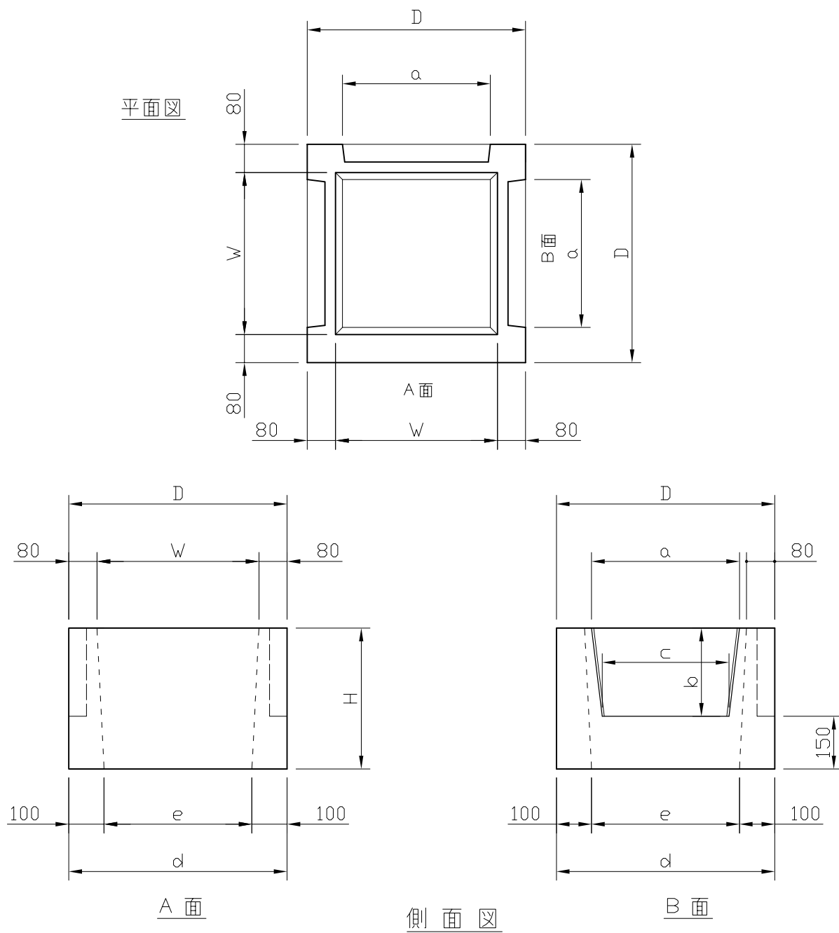
■ 寸法表
