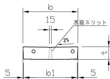
断面図
